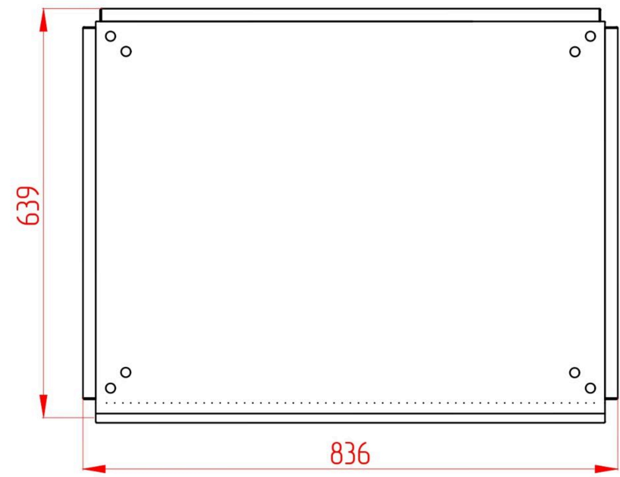
Вид сверху
